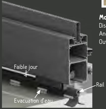
Génie civil avec évacuation d'eau
